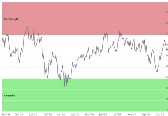
Holdings Above/Below 50 DMA (VWO)
